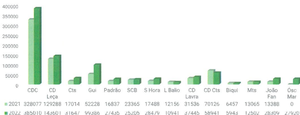
Gráfico 2 – Consumos de eletricidade – Pavilhões e Complexos Desportivos (kWh)
