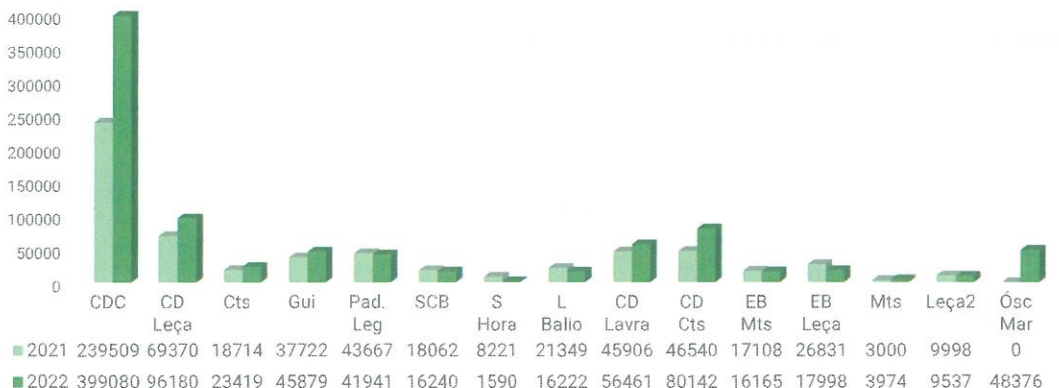
Gráfico 4 – Consumos de gás – Pavilhões e Complexos Desportivos (kWh)
